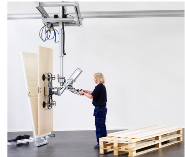
Door gripper
